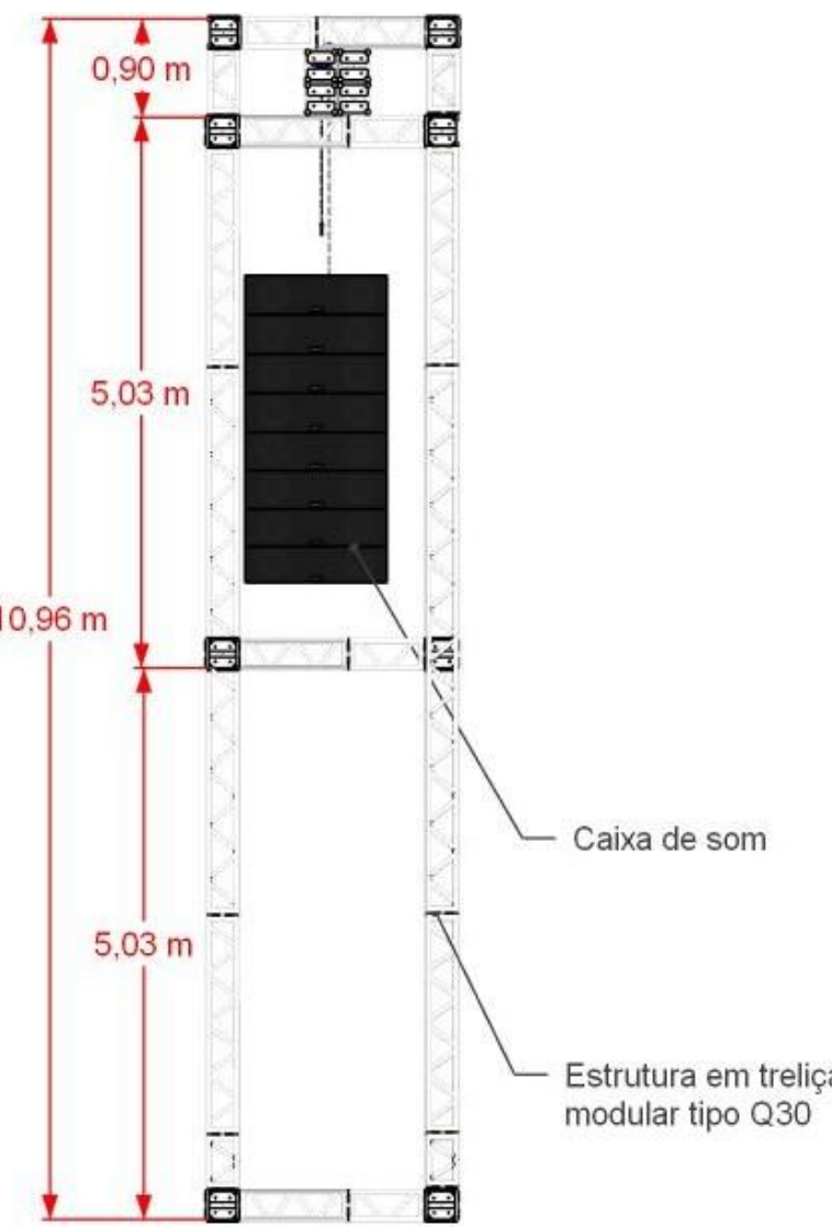
VISTA FRONTAL: ESTRUTURA
