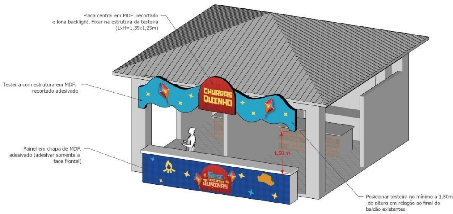
VISTA ISOMÉTRICA
