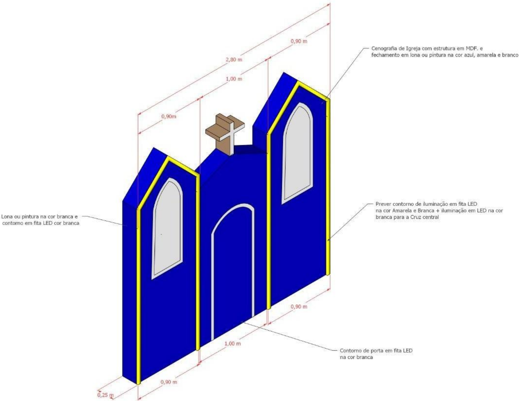
VISTA ISOMÉTRICA
