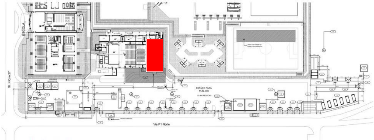
IMPLANTAÇÃO
