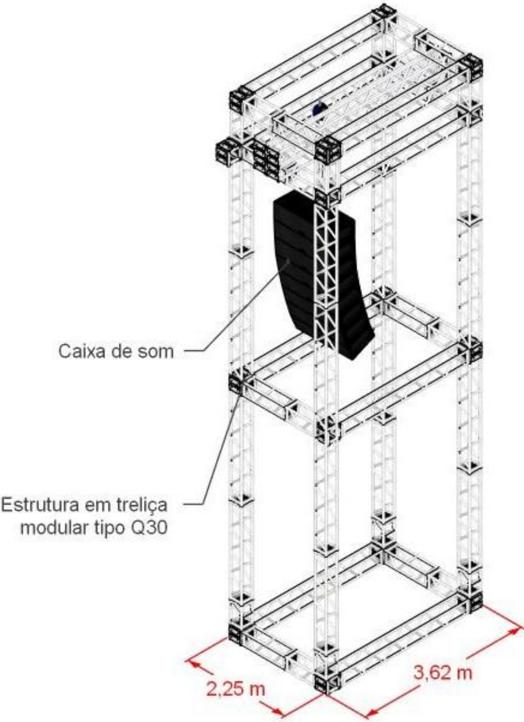
ISOMÉTRICA ESTRUTURA
