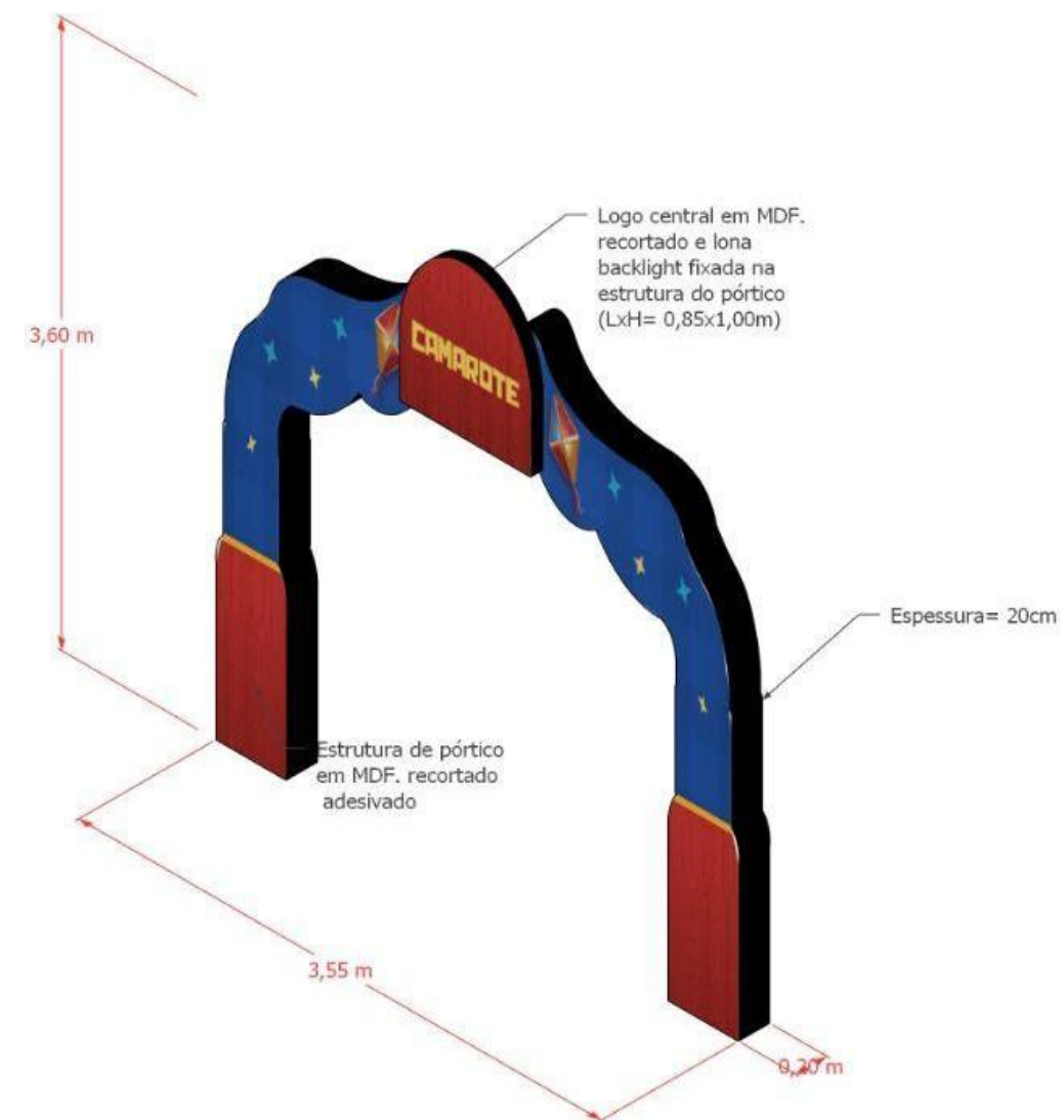
VISTA ISOMÉTRICA
