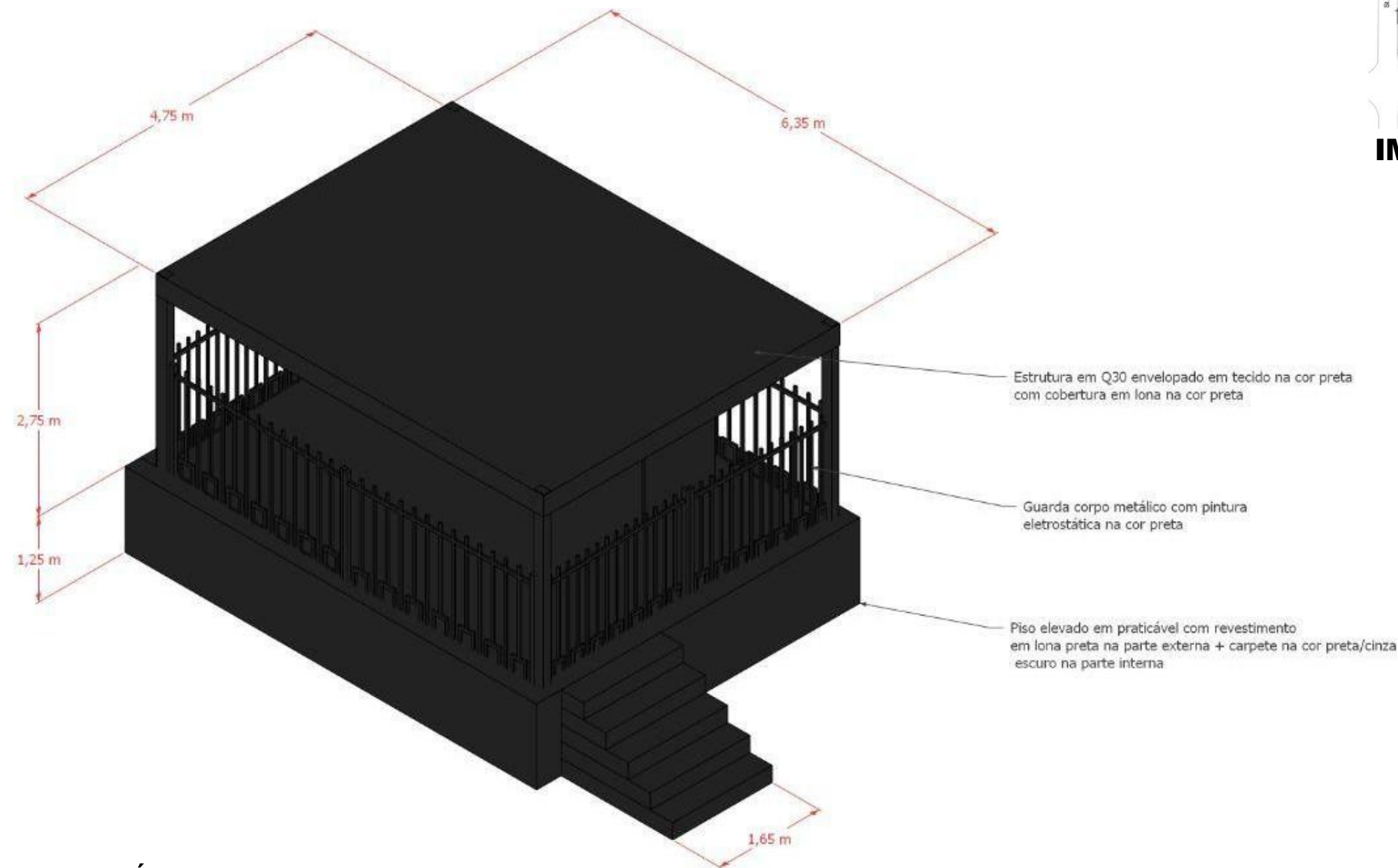
VISTA ISOMÉTRICA: GERAL
