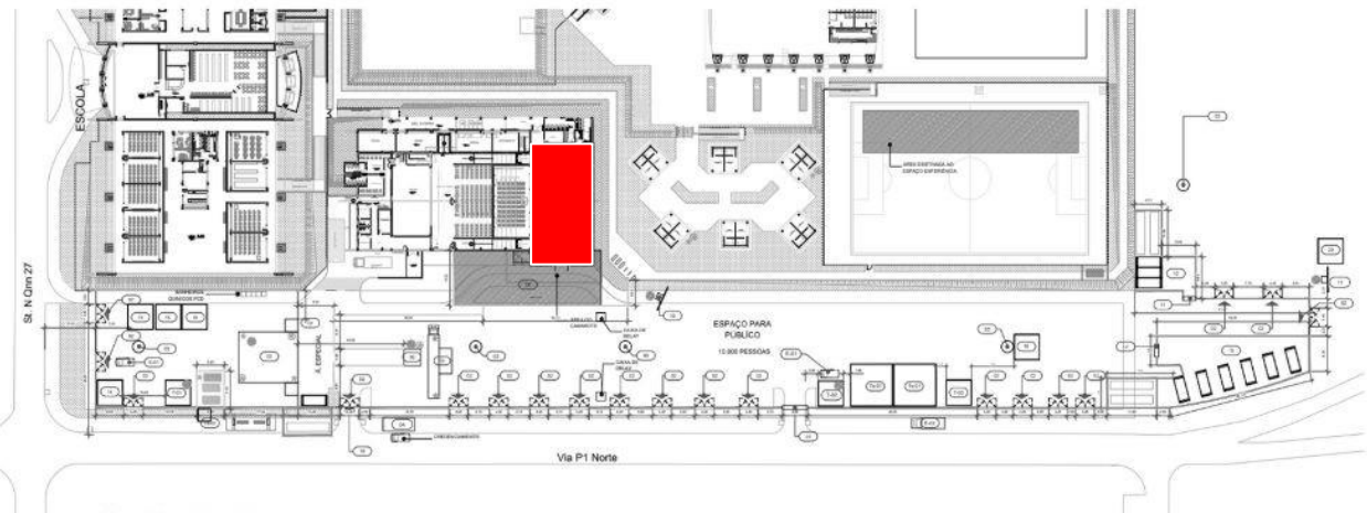
IMPLANTAÇÃO
