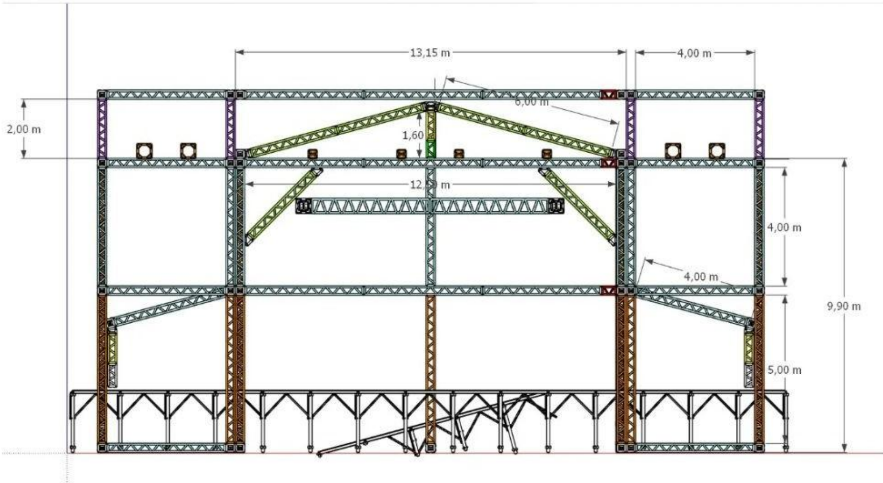
VISTA ESTRUTURA
