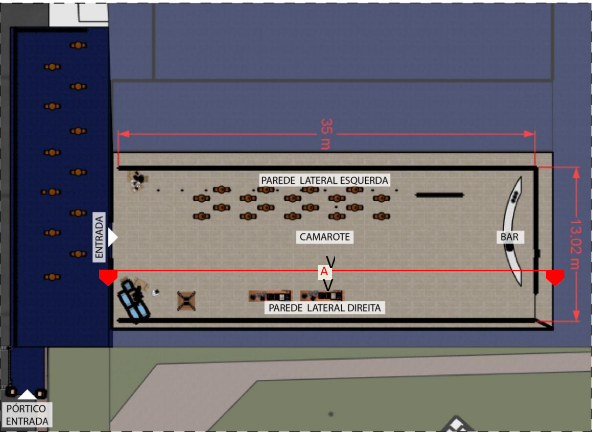
LAYOUT INTERNO
